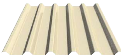
Профилированный лист НС-35х1000-A Толщина материала 0.45 - 0.9 мм
